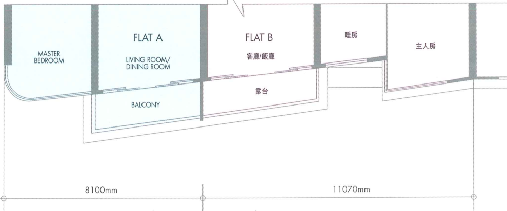
36/F - 38/F PART PLAN 36/F - 38/F 部份平面圖
